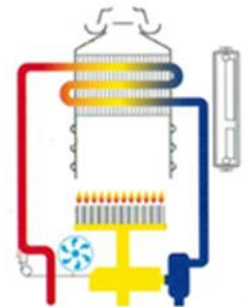
DIAGRAMA FUNCIONAL
